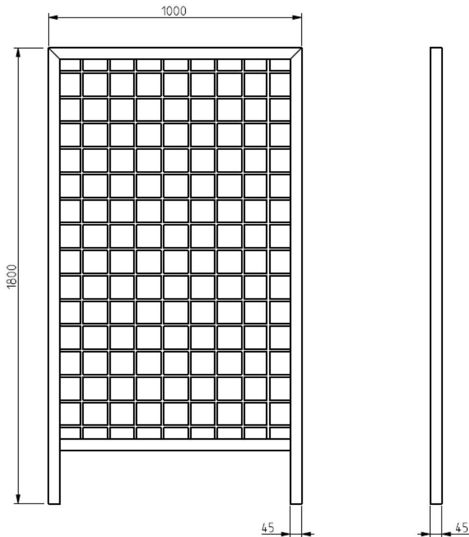
Figur 8: Spaljé infälld i ram och armeringsnät.
