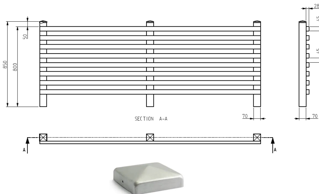
Figur 13: Utformning av staket samt stolphatt.
